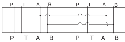
JIS油圧図記号
